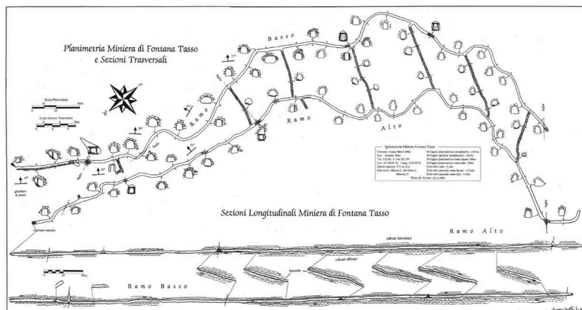
Miniera di Fontana Tasso – Planimetria e sezione
