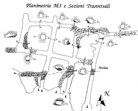
Foto: alcuni degli ingressi e la planimetria della miniera M3
